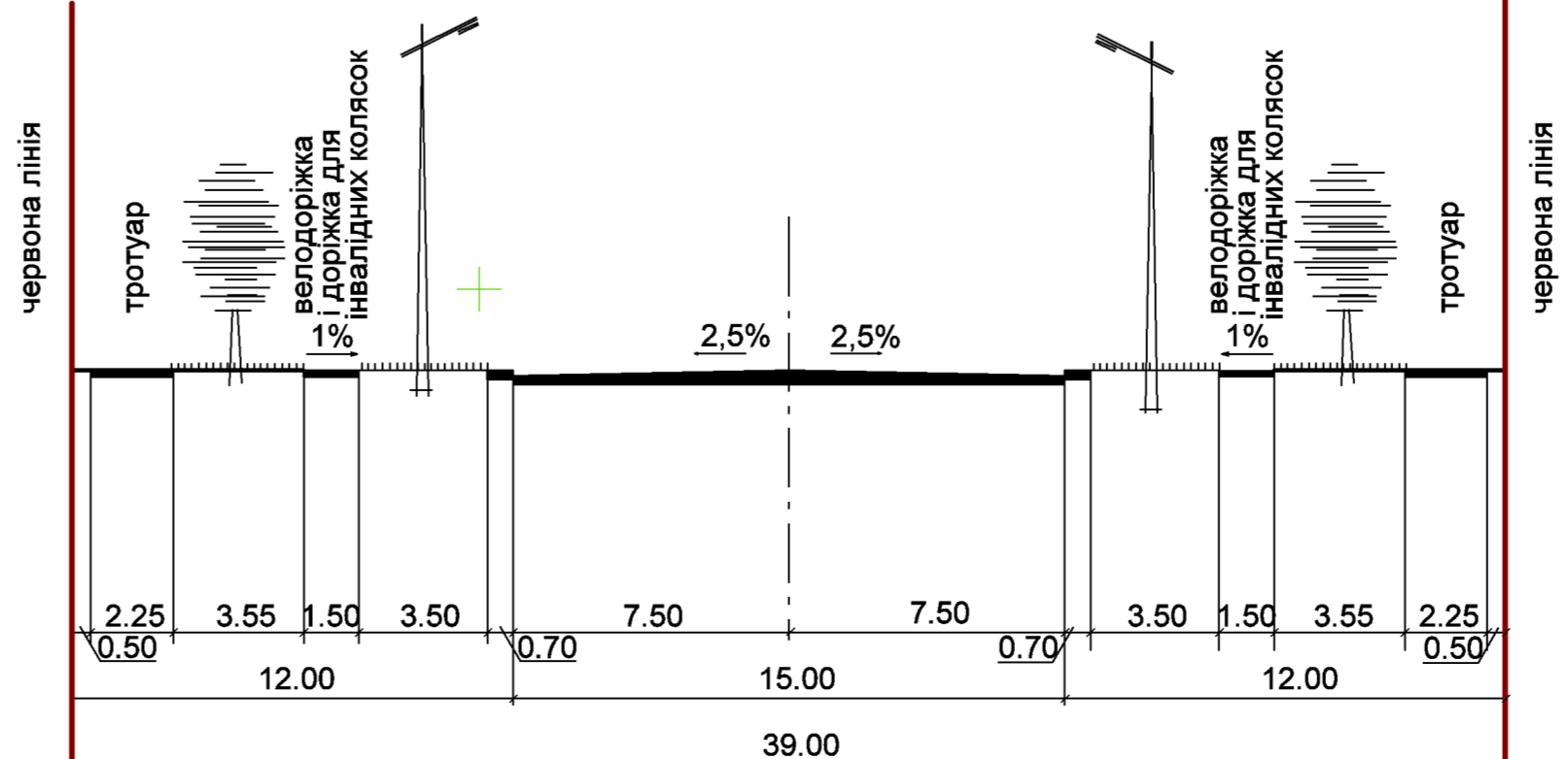
Розріз I-I
