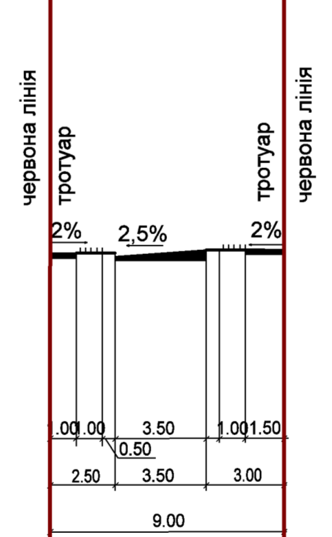
Розріз II-II
